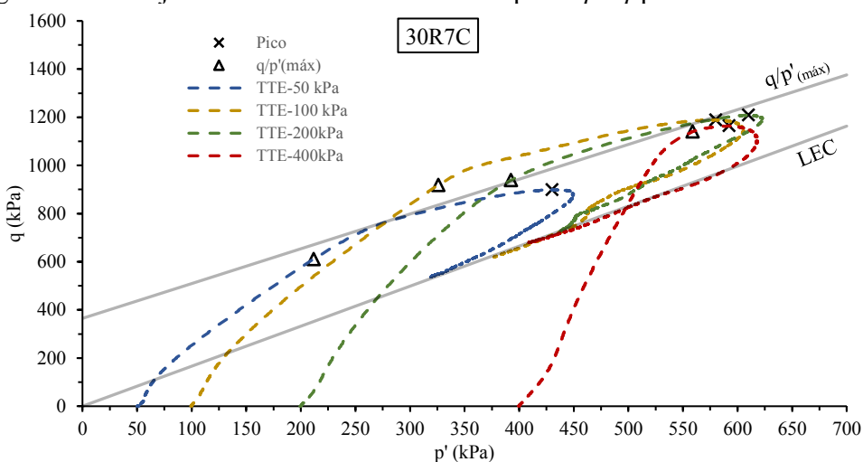
Figura 153 - Trajetórias de tensões efetivas no plano p':q para a amostra 30R7C.
