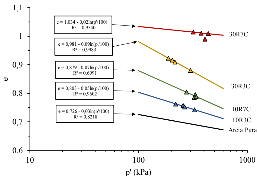
Figura 149 - Linha de estados críticos da areia pura e estabilizada no plano p':e .
