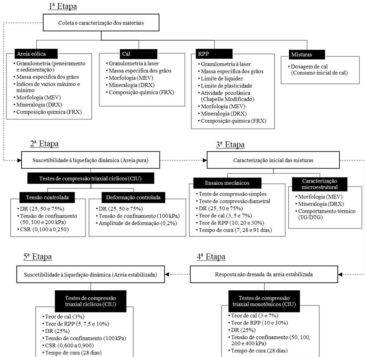
Figura 30 - Esquema do programa experimental da pesquisa.
