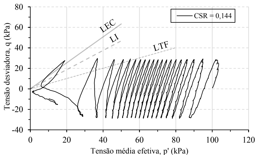
Figura 55 - Trajetória de tensões efetivas para CSR de 0,144.
