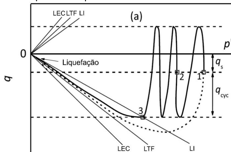
Figura 8 - Relação entre resposta cíclica e monotônica de uma areia fofa.
