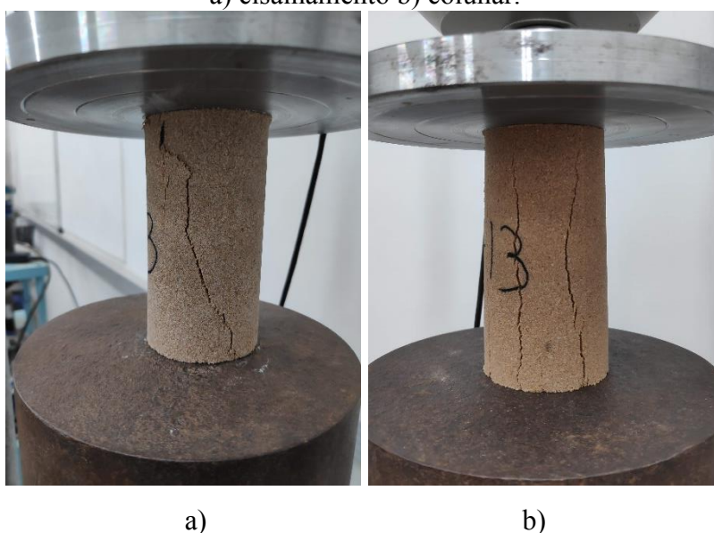
Figura 116 - Modos de ruptura da areia estabilizada em ensaios de compressão não confinada. a) cisalhamento b) colunar.
