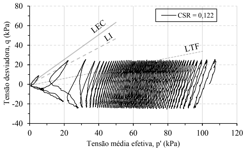
Figura 54 - Trajetória de tensões efetivas para CSR de 0,122.
