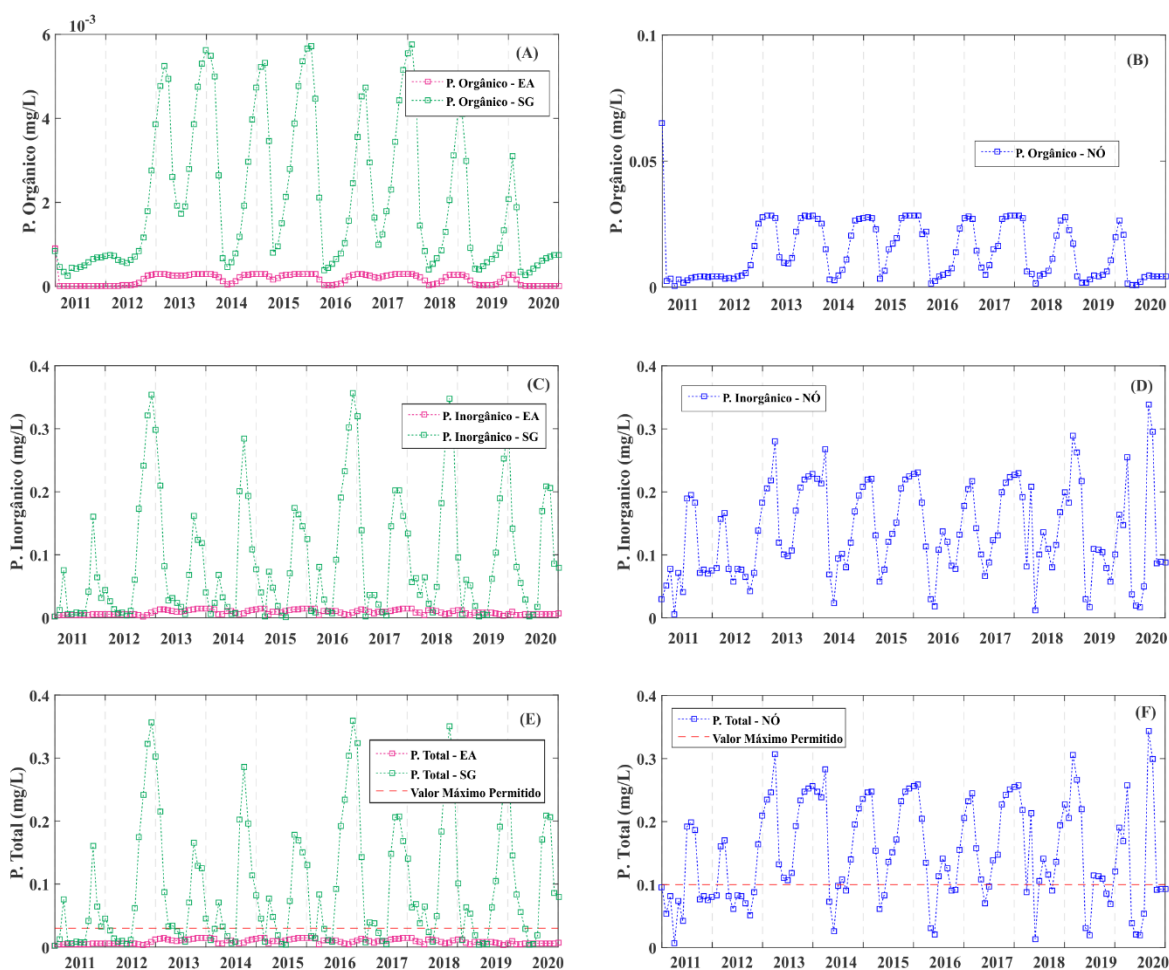
Figura 33 – Concentrações de fósforo orgânico, inorgânico e total nos reservatórios Engenheiro Ávidos, São Gonçalo e no nó, considerando o lançamento de esgotos brutos e dos efluentes agrícolas no Cenário C1.
