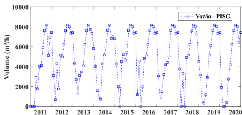
Figura 35 – Vazões destinadas ao atendimento do PISG para o Cenário C2.
