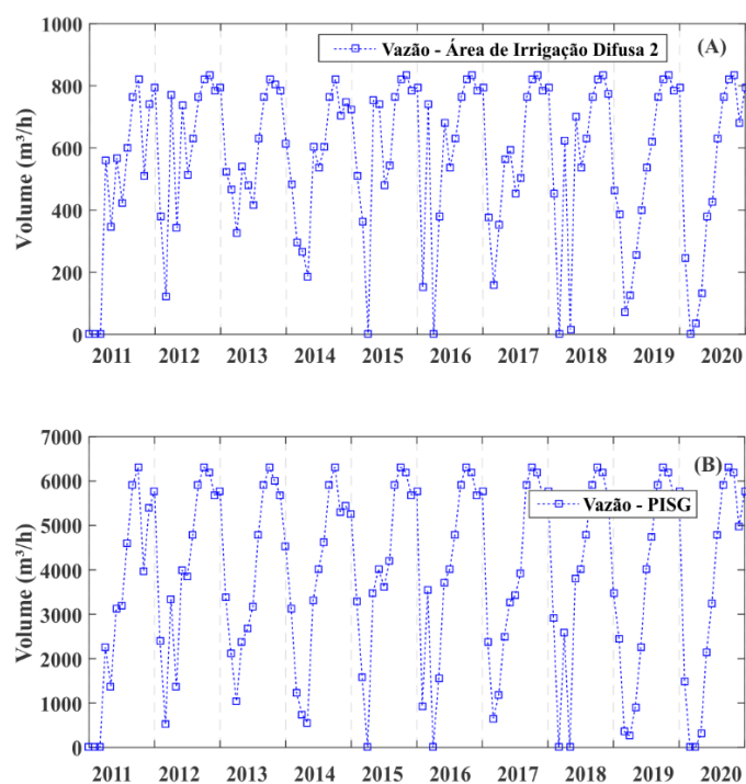
Figura 49 – Vazões destinadas ao atendimento da área de irrigação difusa 2 (A) e do PISG (B) para o Cenário C4.
