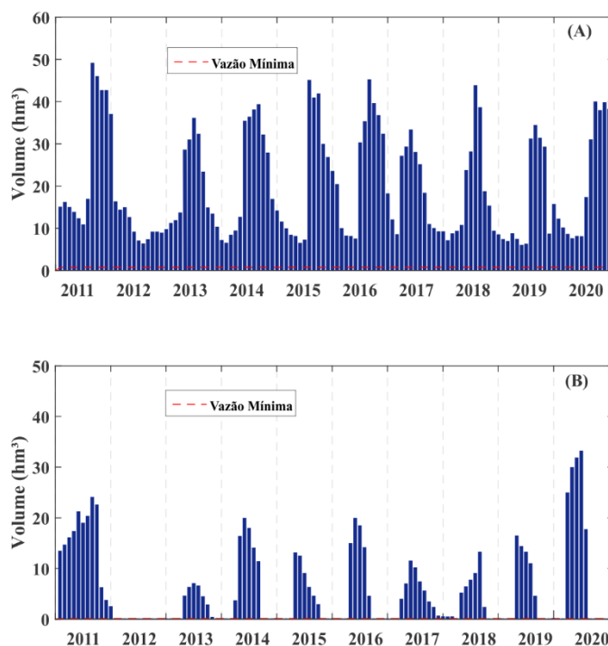
Figura 37 – Volumes defluentes dos reservatórios Engenheiro Ávidos (A) e São Gonçalo (B) para o Cenário C2.
