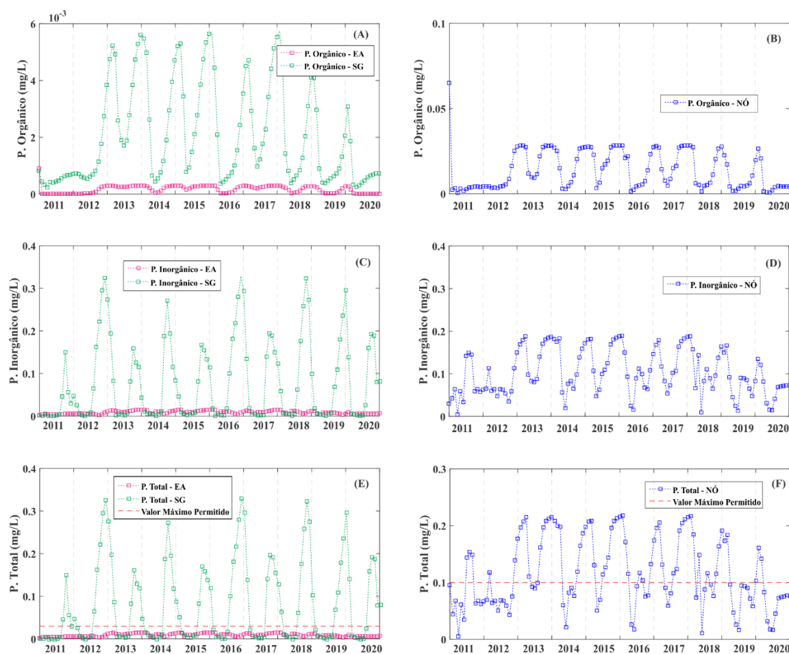
Figura 32 – Concentrações de fósforo orgânico, inorgânico e total nos reservatórios Engenheiro Ávidos, São Gonçalo e no nó, considerando o lançamento de esgotos brutos no Cenário C1.
