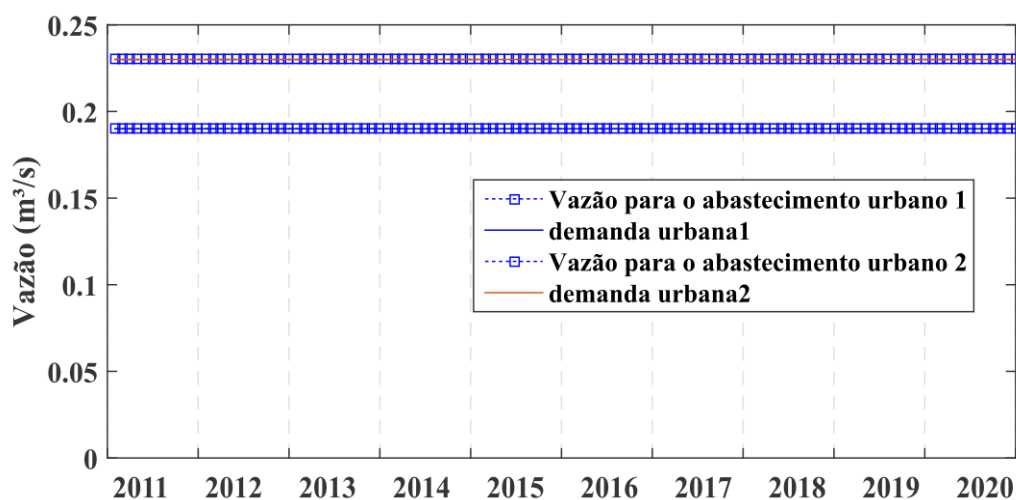
Figura 23 – Abastecimento urbano do município de Cajazeiras (abastecimento urbano 1) e dos municípios de Sousa, Marizópolis e Nazarezinho (abastecimento urbano 2) – Cenário C1
