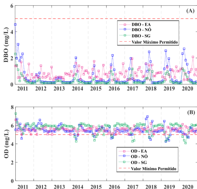
Figura 45 – Concentrações de DBO (A) e OD (B) para os reservatórios e o nó no Cenário C3.
