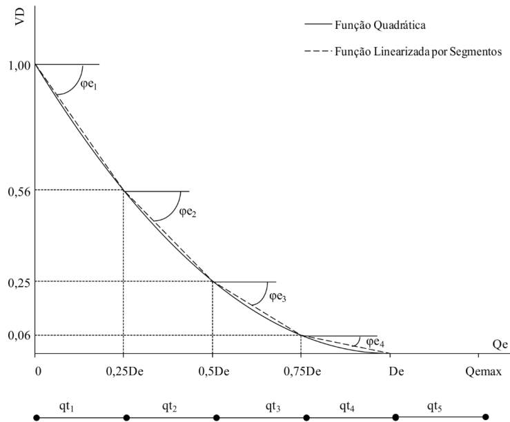
Figura 8 – Função objetivo linearizada correspondente ao volume defluente dos reservatórios.
