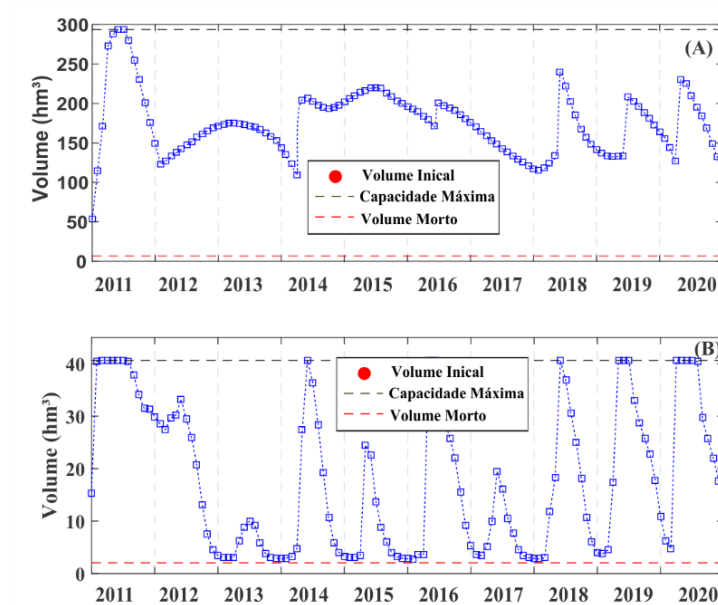
Figura 26 – Volume dos reservatórios Engenheiro Ávidos (A) e São Gonçalo (B) para o Cenário C1.
