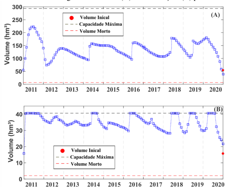
Figura 36 – Volume dos reservatórios Engenheiro Ávidos (A) e São Gonçalo (B) para o Cenário C2.
