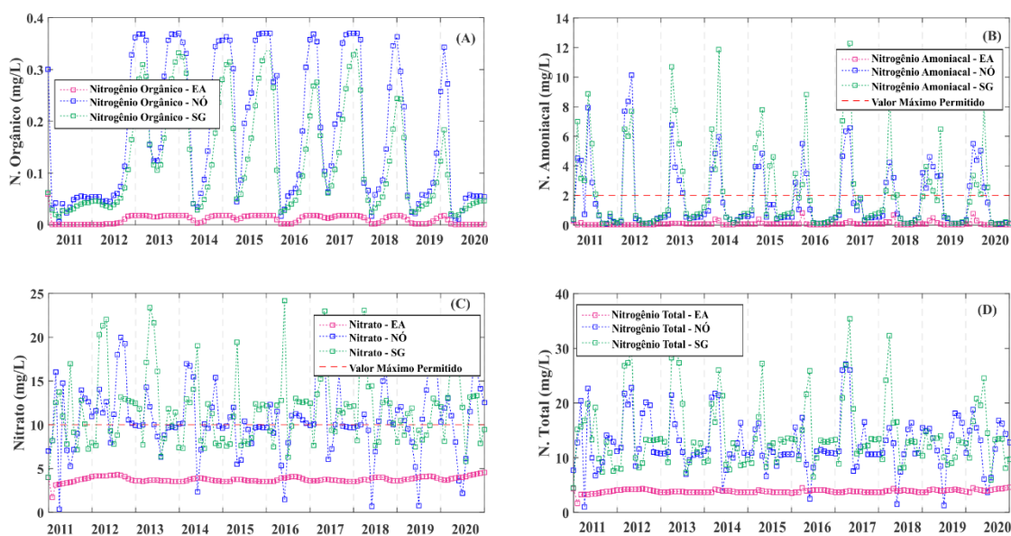
Figura 31 – Concentrações de nitrogênio orgânico (A), amoniacal (B), nitrato (C) e nitrogênio total (D) nos reservatórios Engenheiro Ávidos, São Gonçalo e no nó, considerando o lançamento de esgotos brutos e dos efluentes agrícolas no Cenário C1.
