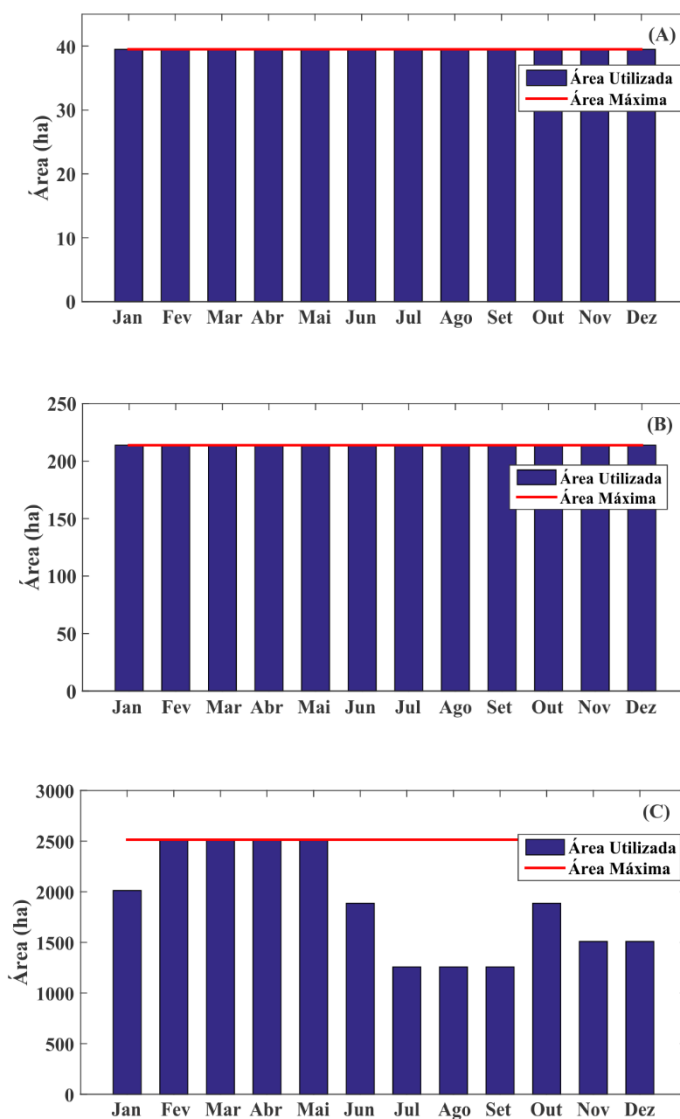
Figura 24 – Áreas médias cultivadas para a irrigação difusa 1 (A), 2 (B) e o PISG (C) – Cenário C1.
