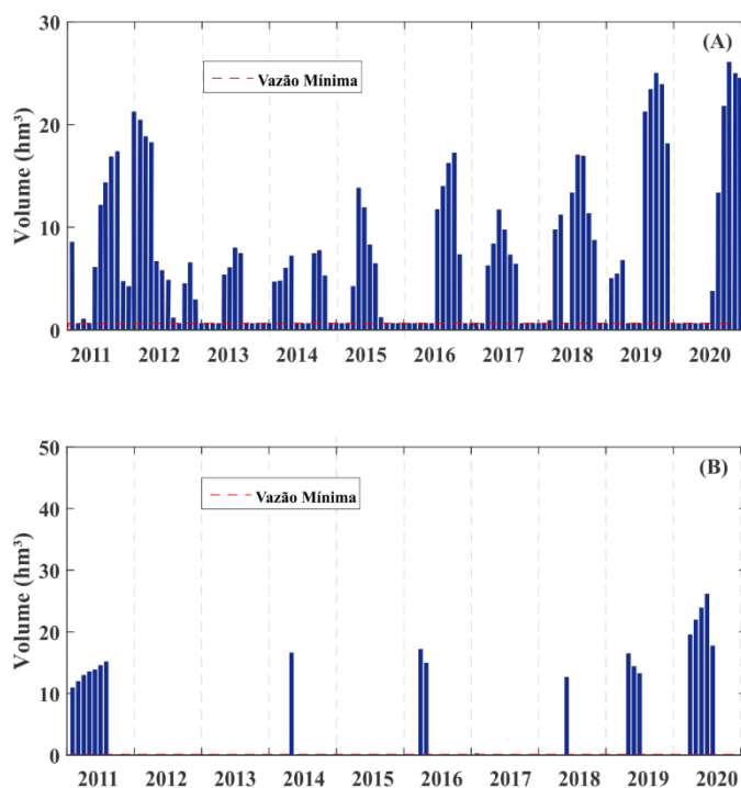
Figura 27 – Volumes defluentes dos reservatórios Engenheiro Ávidos (A) e São Gonçalo (B) para o Cenário C1.
