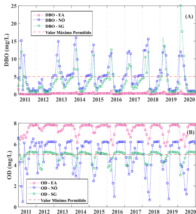
Figura 28 – Concentrações de DBO (A) e OD (B) nos reservatórios Engenheiro Ávidos, São Gonçalo e no nó, considerando o lançamento de esgotos brutos no Cenário C1.
