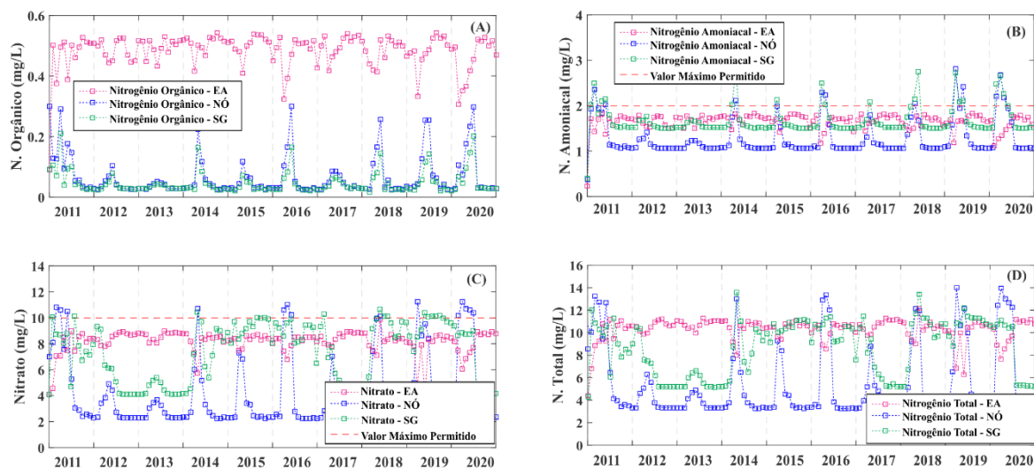
Figura 53 – Concentrações de nitrogênio orgânico (A), amoniacal (B), nitrato (C) e total (D) para os reservatórios e o nó no Cenário C4.
