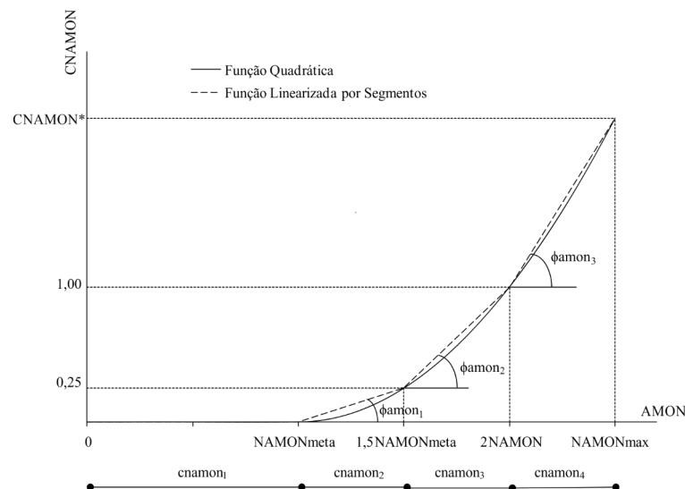
Figura 16 – Gráfico da função objetivo quadrática linearizada por segmentos da q -ézima concentração de NAMON para um mês t .
