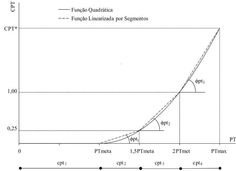
Figura 15 – Gráfico da função objetivo quadrática linearizada por segmentos da p -ésima concentração de PT para um mês t .
