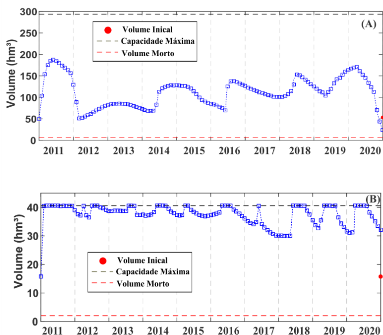
Figura 43 – Volume dos reservatórios Engenheiro Ávidos (A) e São Gonçalo (B) para o Cenário C3.
