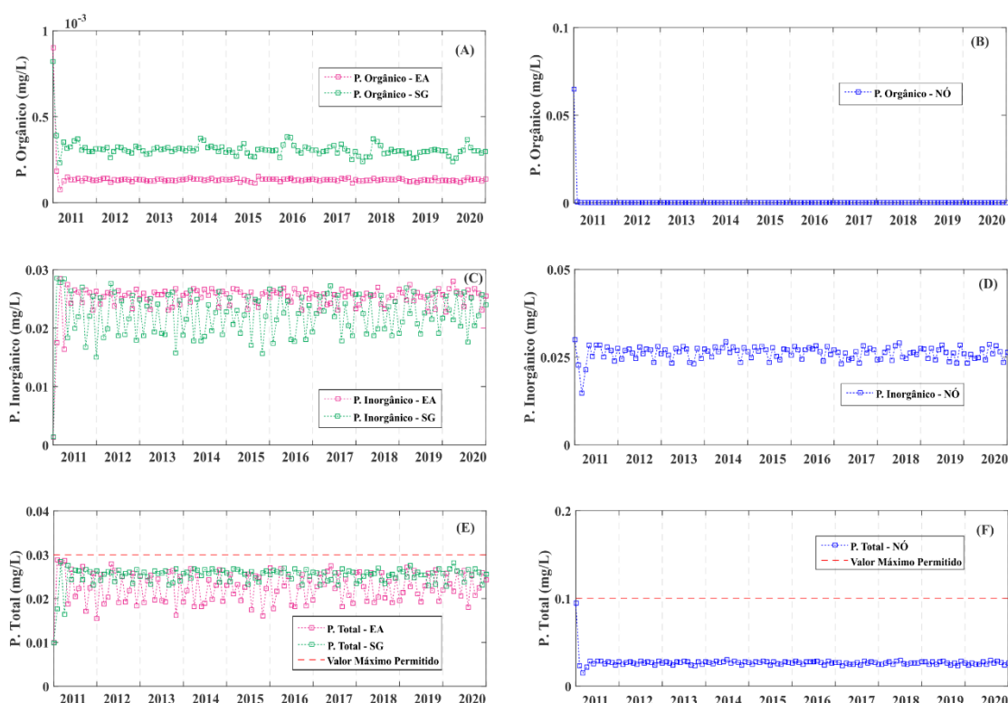
Figura 40 – Concentrações de fósforo orgânico, inorgânico e total para os reservatórios e o nó no Cenário C2.
