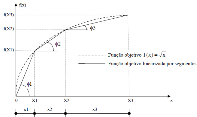
Figura 1 – Função objetivo não-linear e linearizada pelo artifício de linearização por segmentos.
