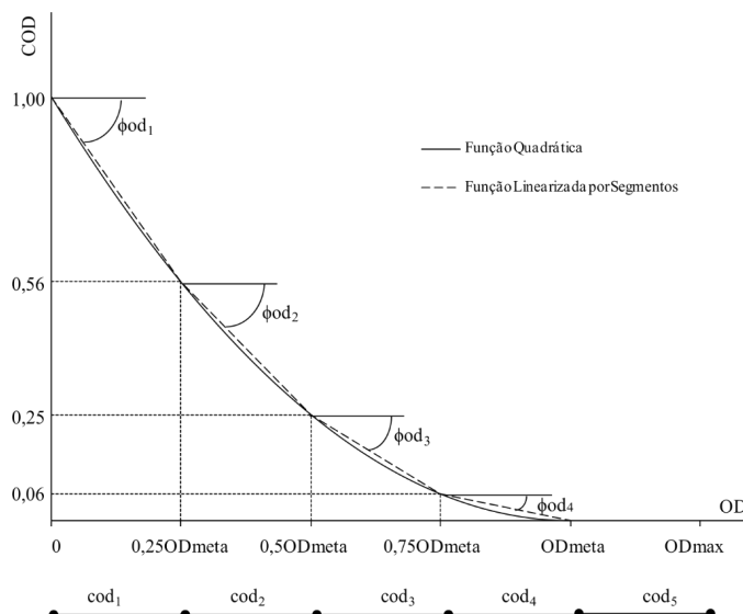
Figura 14 – Gráfico da função objetivo quadrática linearizada por segmentos da v -ézima concentração de OD para um mês t .
