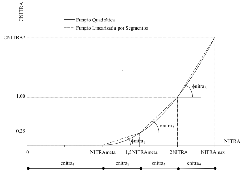
Figura 17 – Gráfico da função objetivo quadrática linearizada por segmentos da x -ézima concentração de NITRA para um mês t .
