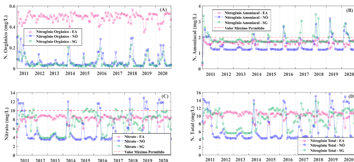
Figura 46 – Concentrações de nitrogênio orgânico (A), amoniacal (B), nitrato (C) e total (D) para os reservatórios e o nó no Cenário C3.
