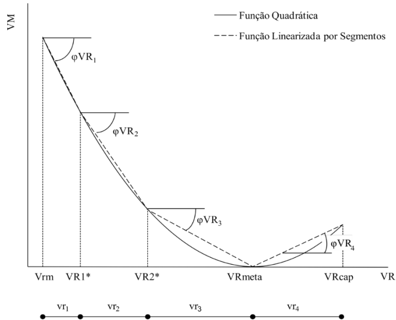
Figura 9 – Função objetivo linearizada correspondente ao volume dos reservatórios.
