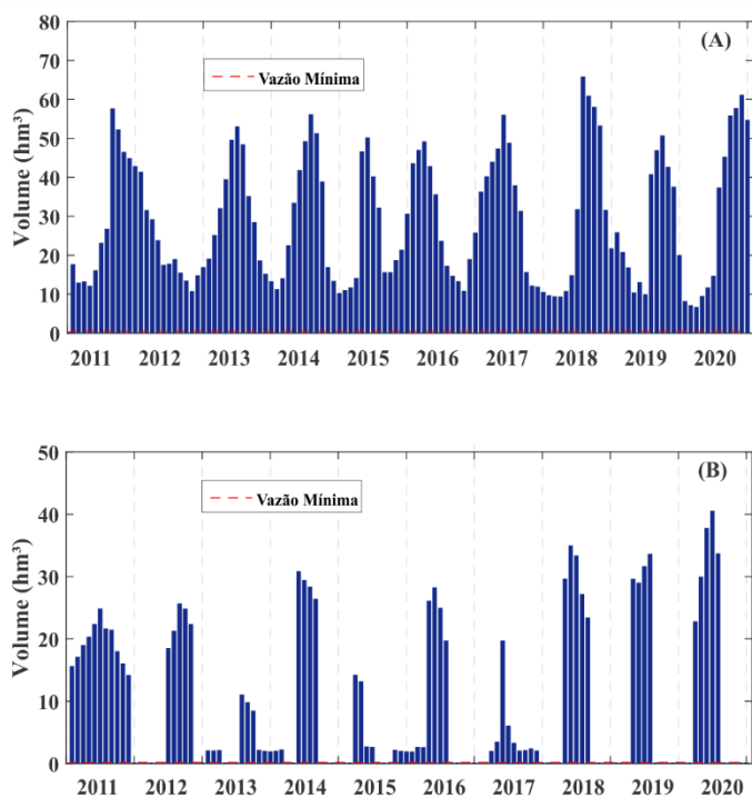
Figura 51 – Volumes defluentes dos reservatórios Engenheiro Ávidos (A) e São Gonçalo (B) para o Cenário C4.
