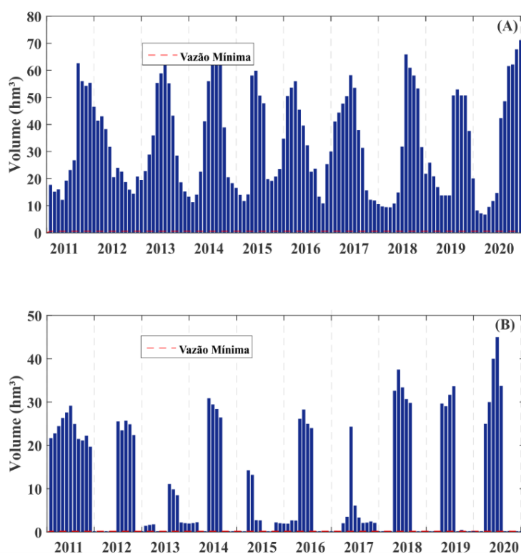
Figura 44 – Volumes defluentes dos reservatórios Engenheiro Ávidos (A) e São Gonçalo (B) para o Cenário C3.
