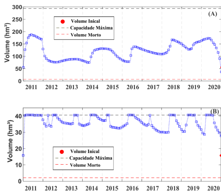
Figura 50 – Volume dos reservatórios Engenheiro Ávidos (A) e São Gonçalo (B) para o Cenário C4.
