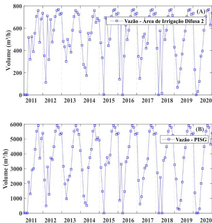
Figura 42 – Vazões destinadas ao atendimento da área de irrigação difusa 2 (A) e o PISG (B) para o Cenário C3.
