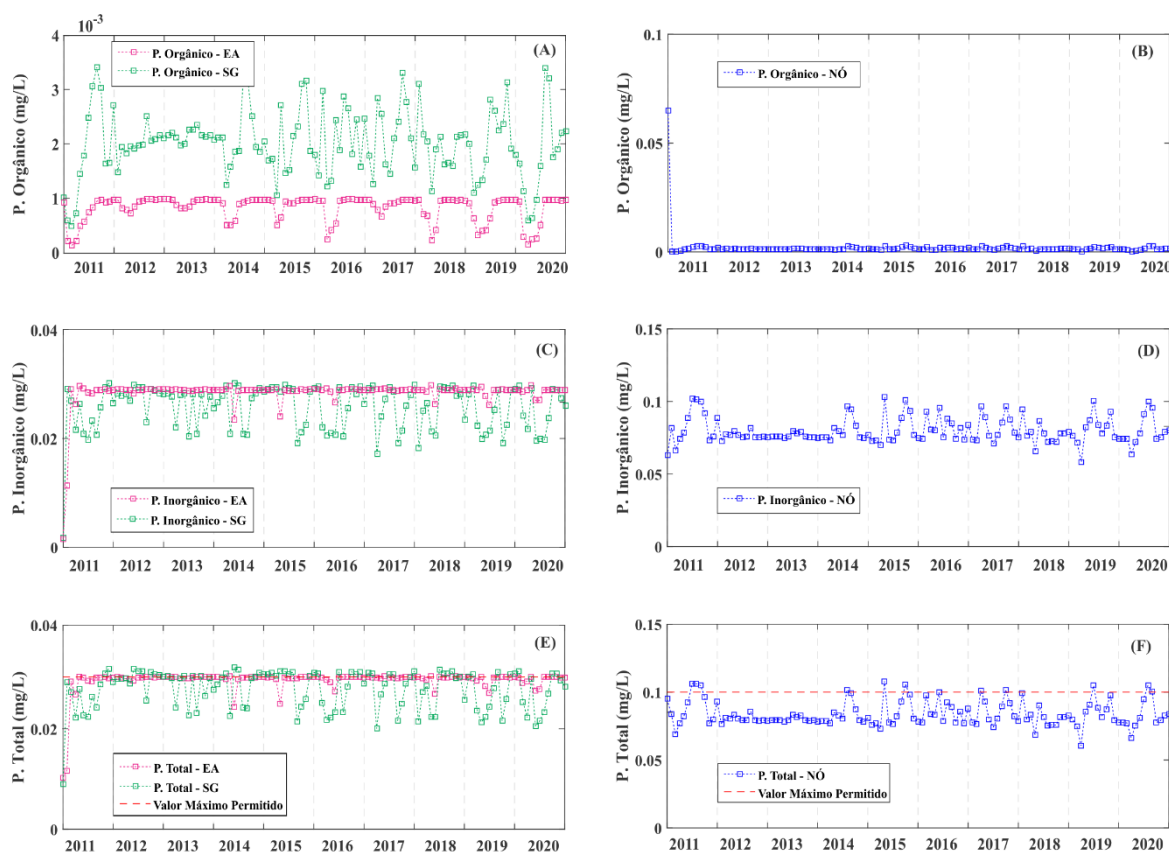
Figura 47 – Concentrações de fósforo orgânico, inorgânico e total para os reservatórios e o nó no Cenário C3.
