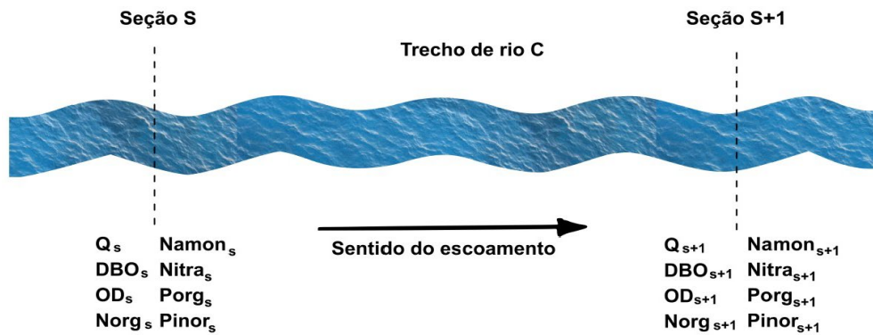
Figura 12 – Diagrama representando os componentes avaliados pelo modelo no processo de autodepuração ao longo do trecho do rio.
