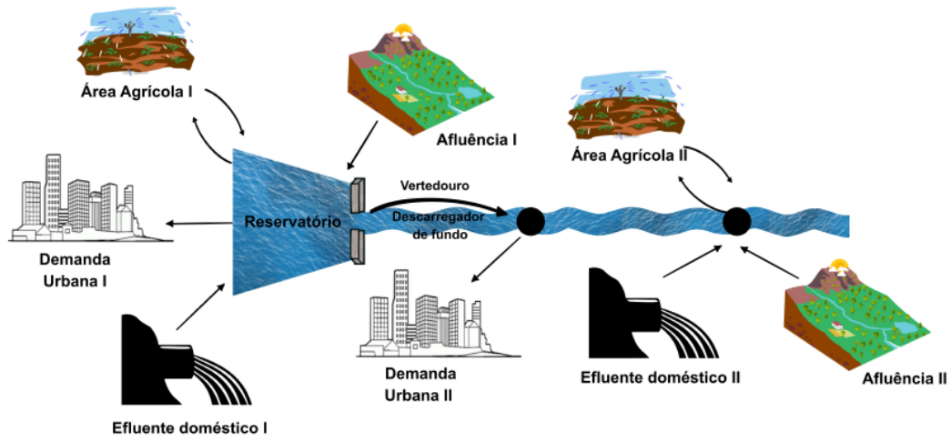
Figura 10 – Representação esquemática do reservatório e seus componentes no modelo de otimização.
