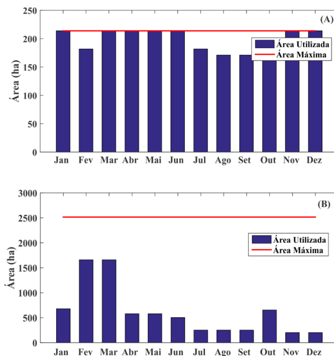
Figura 48 – Áreas médias cultivadas para a irrigação difusa 2 (A) e o PISG (B) – Cenário C4.
