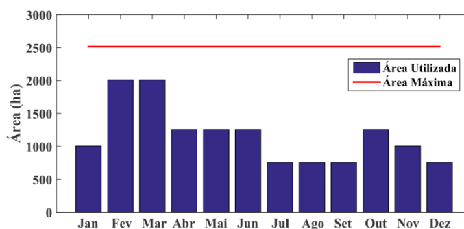
Figura 34 – Áreas médias cultivadas no PISG – Cenário C2.
