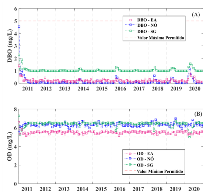
Figura 38 – Concentrações de DBO (A) e OD (B) para os reservatórios e o nó no Cenário C2.
