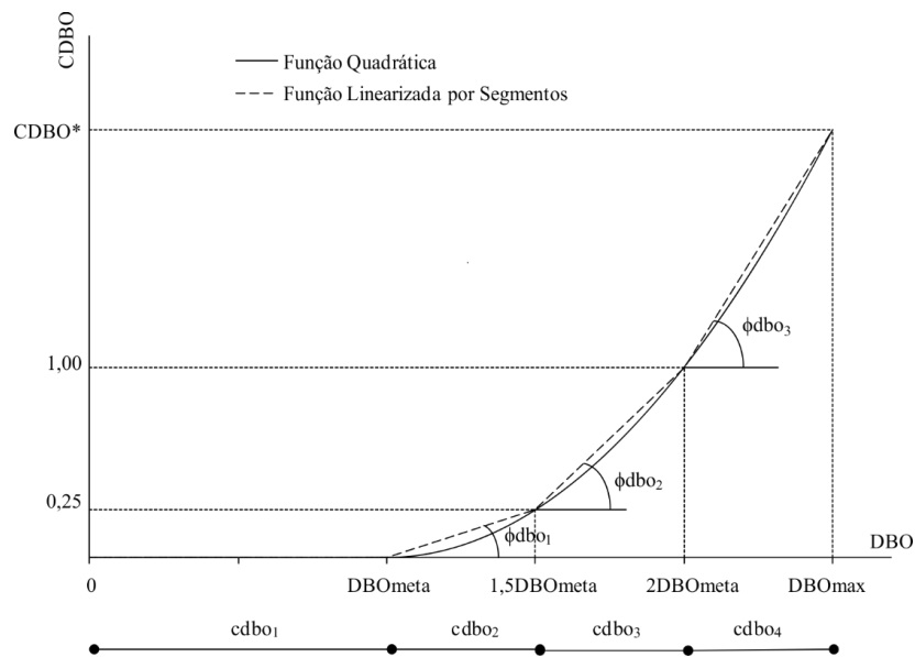
Figura 13 – Gráfico da função objetivo quadrática linearizada por segmentos da \mu -ézima concentração de DBO para um mês t .
