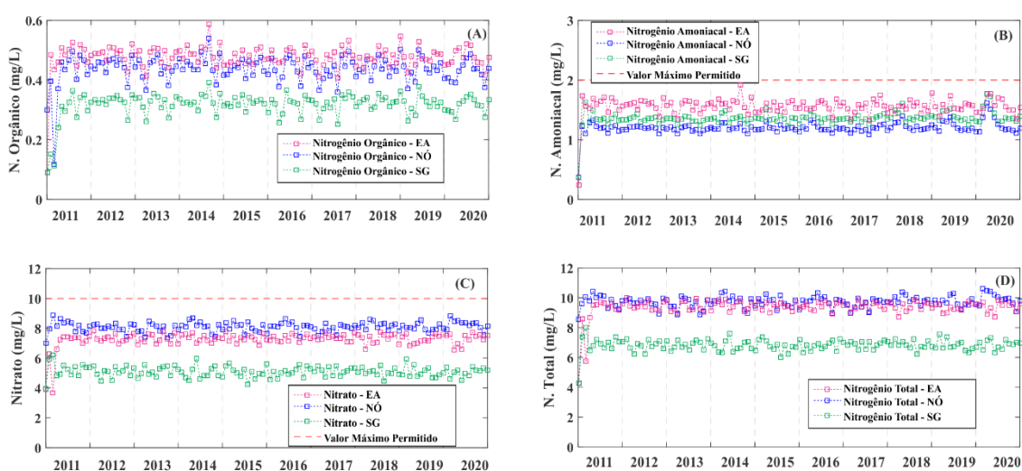
Figura 39 – Concentrações de nitrogênio orgânico (A), amoniacal (B), nitrato (C) e total (D) para os reservatórios e o nó no Cenário C2.
