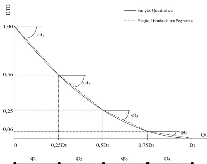
Figura 7 – Função objetivo linearizada correspondente ao volume destinado ao atendimento das demandas.
