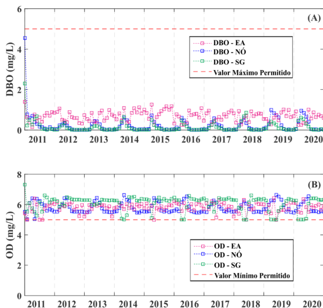
Figura 52 – Concentrações de DBO (A) e OD (B) para os reservatórios e o nó no Cenário C4
