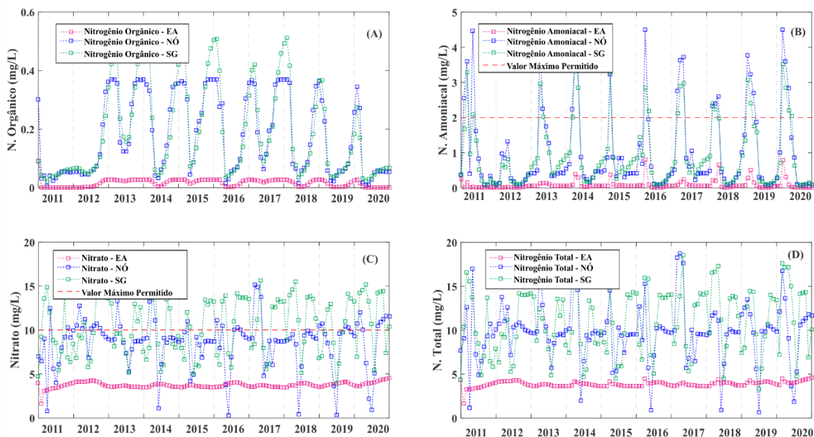
Figura 30 – Concentrações de nitrogênio orgânico (A), amoniacal (B), nitrato (C) e nitrogênio total (D) nos reservatórios Engenheiro Ávidos, São Gonçalo e no nó, considerando o lançamento de esgotos brutos no Cenário C1.
