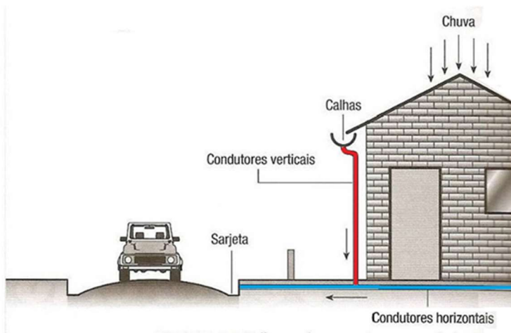
Figura 3 - Calhas e Condutores do SAAC
