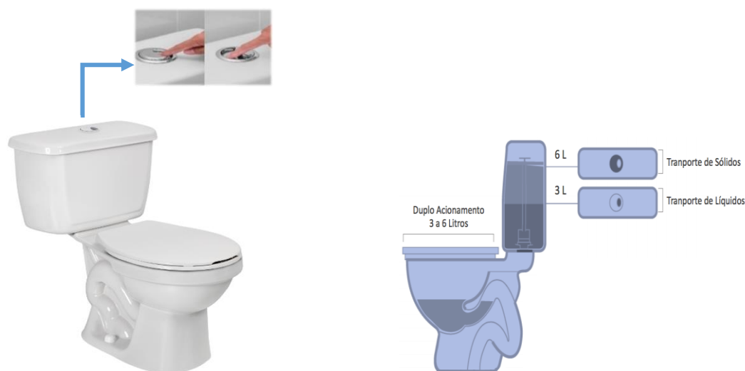
Figura 6 - Bacia sanitária de acionamento duplo.
