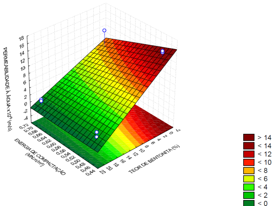
Figura 35: Superfície resposta do DCC para Energia de compactação x Teor de bentonita – permeabilidade à água
