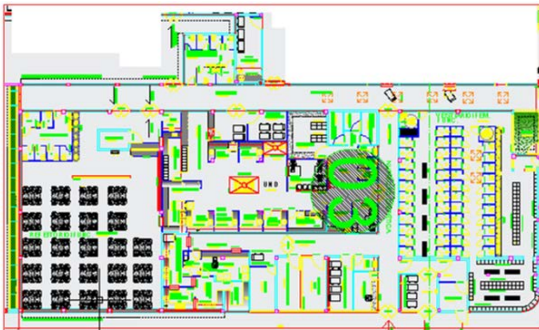
Figura 3.8 – Apoio técnico do Hospital Regional de Emergência e Trauma Dom Luís Gonzaga Fernandes.
