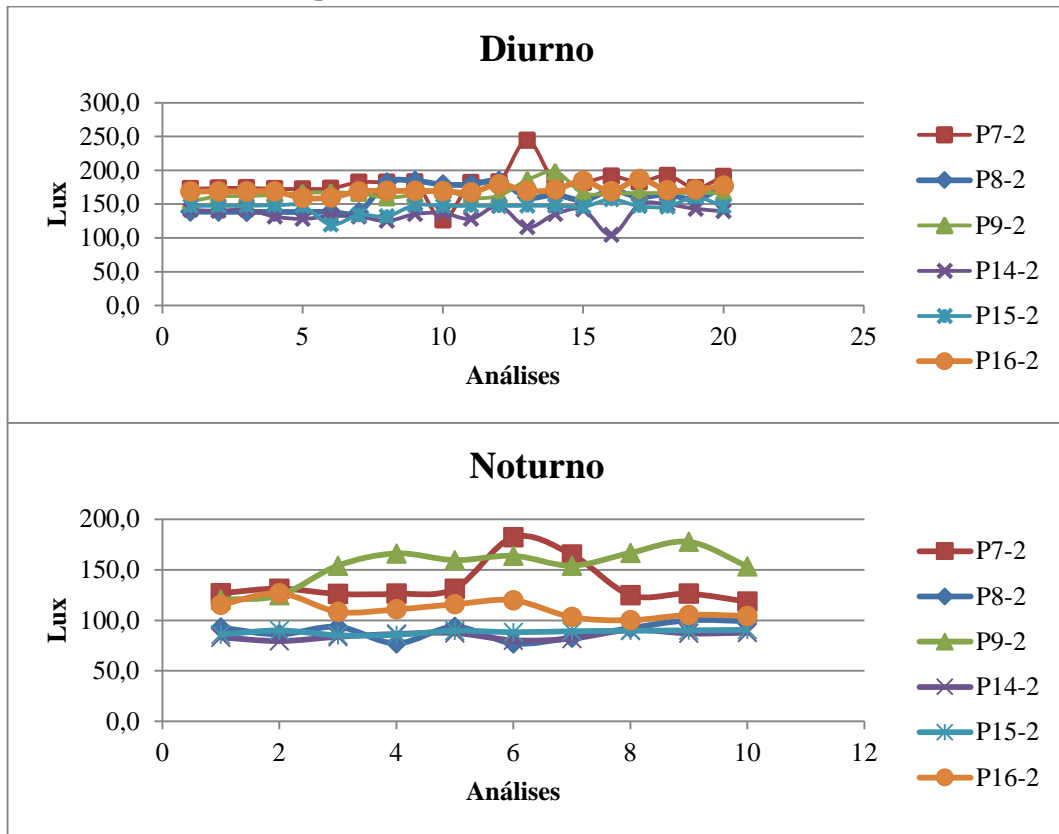
Figura 4.12 – Iluminâncias aferidas nas salas de enfermagem das enfermarias P7-2, P8-2, P9-2, P14-2, P15-2 e P16-2 no período diurno (a) e noturno (b).
