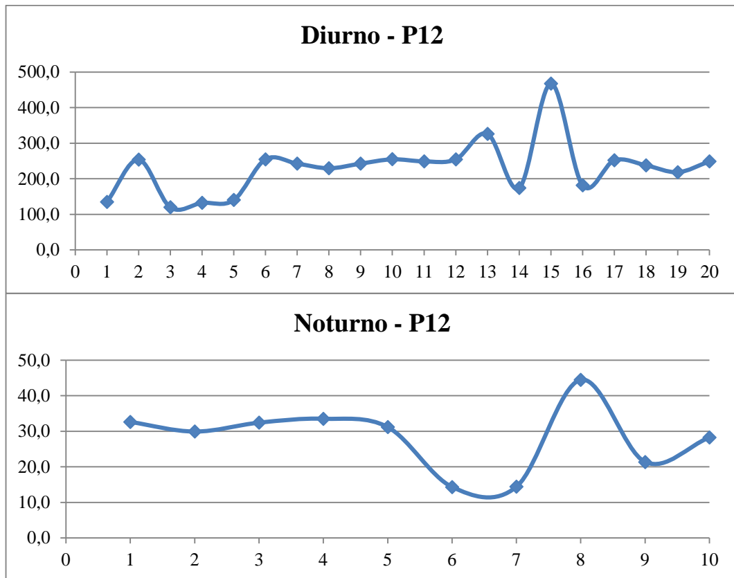
Figura 4.22 – Níveis de iluminação aferidos na sala da coordenação de estágio nos períodos diurno e noturno.
