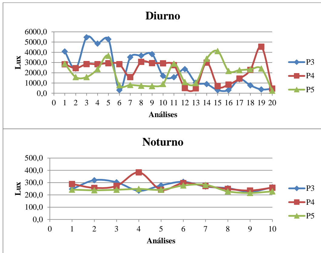
Figura 4.6 – Iluminâncias nos Pontos P3, P4 e P5 localizados em corredores.
