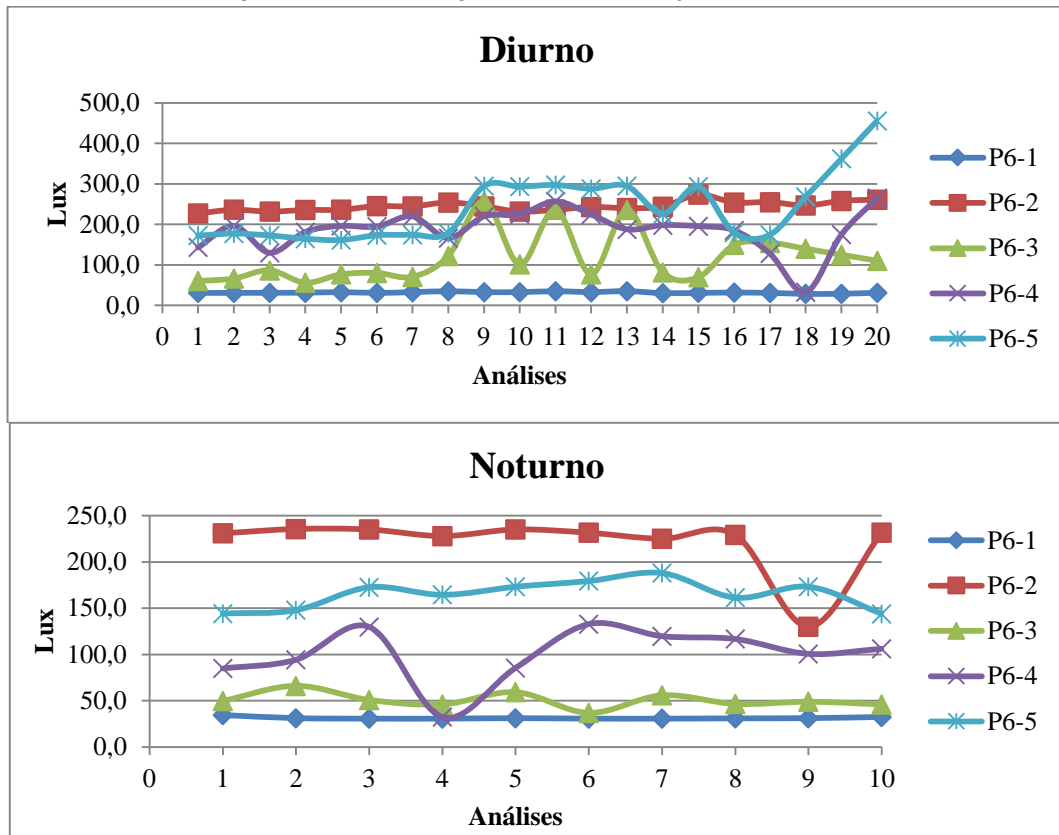
Figura 4.8 – Iluminâncias aferidas no setor da lavanderia (P6): P6-1 entrada, P6-2 mesa de separação, P6-3 centrífuga, P6-4 armazenagem e P6-5 área suja.
