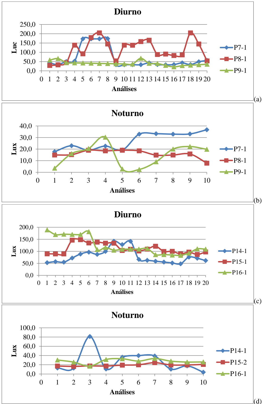
Figura 4.10 – Aferição das iluminâncias no corredor central de acesso às enfermarias: pavimento térreo P7-1, P8-1 e P9-1 diurno (a) e noturno (b); primeiro pavimento P14-1, P15-1, P16-1 diurno (c) e noturno (d).
