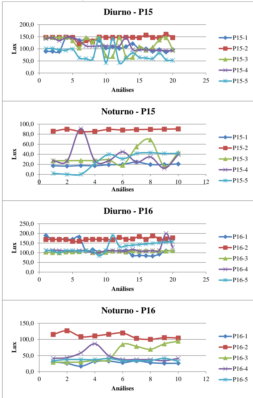
Figura 4.16 – Iluminâncias nos leitos das enfermarias nos pontos P15 e P16: (a) leitos do lado direito e (b) leitos do lado esquerdo.
