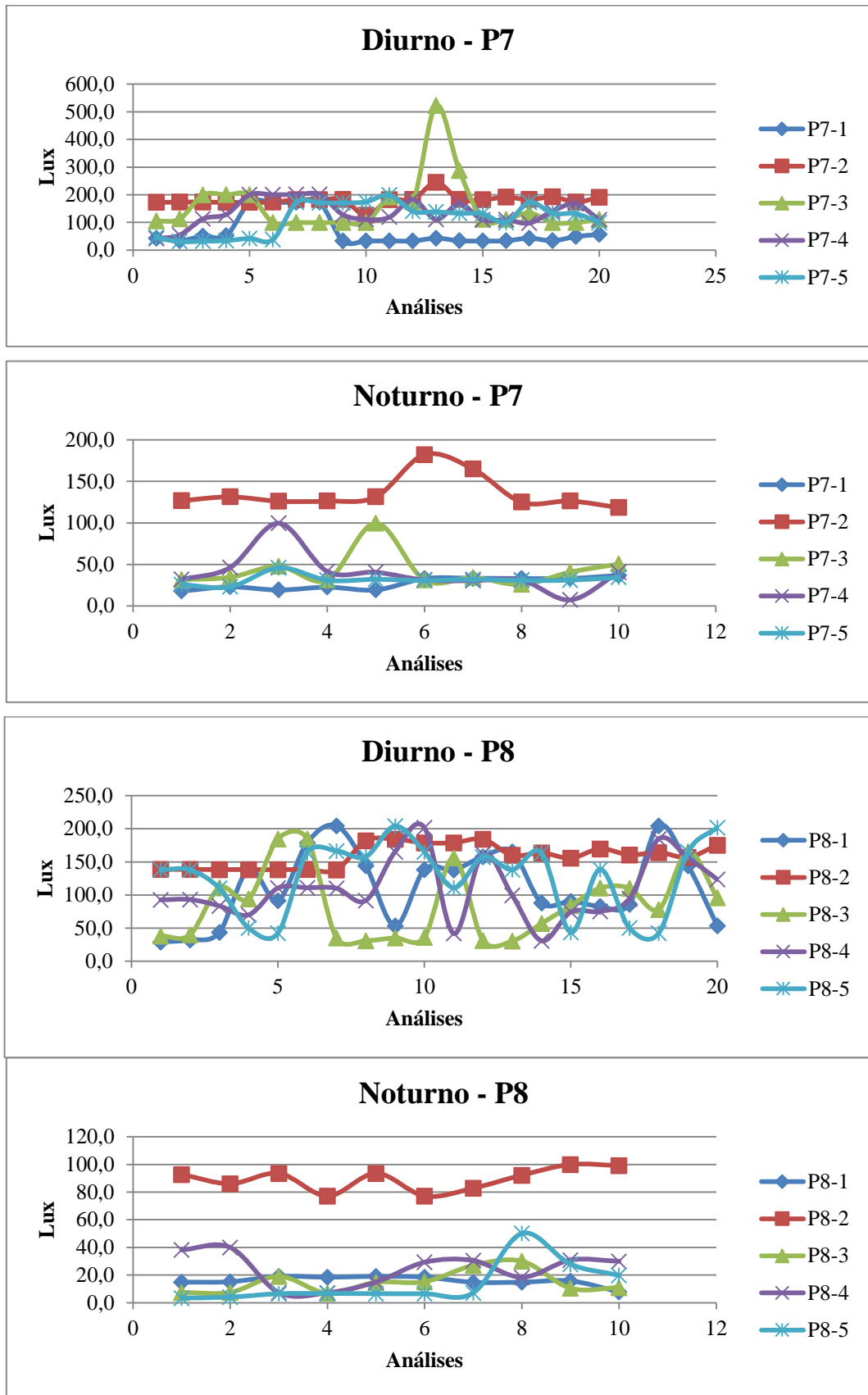
Figura 4.14 – Iluminâncias nos leitos das enfermarias nos pontos P7 e P8: (a) leitos do lado direito e (b) leitos do lado esquerdo.
