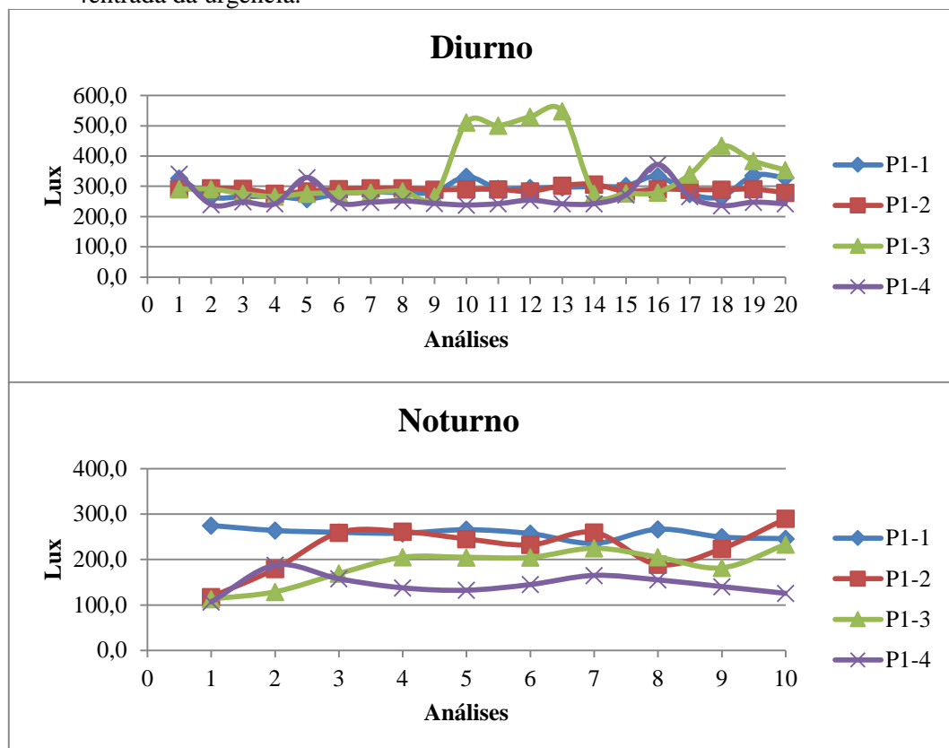
Figura 4.2 – Iluminâncias no setor de pronto atendimento nos turnos dia e noite: P1-1recepção geral dos atendimentos, P1-2 final da recepção, P1-3entrada do setor de emergência eP1-4entrada da urgência.
