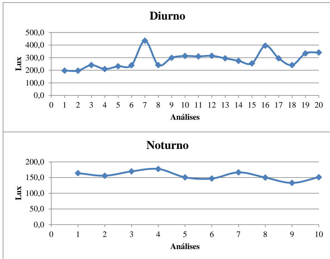
Figura 4.4 – Iluminâncias no setor da área vermelha (P2): (a) diurno e (b) noturno.
